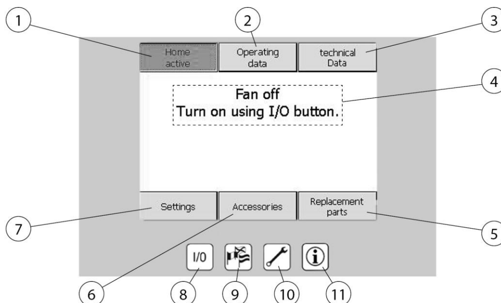
Rys. 38: Elementy obsługi
