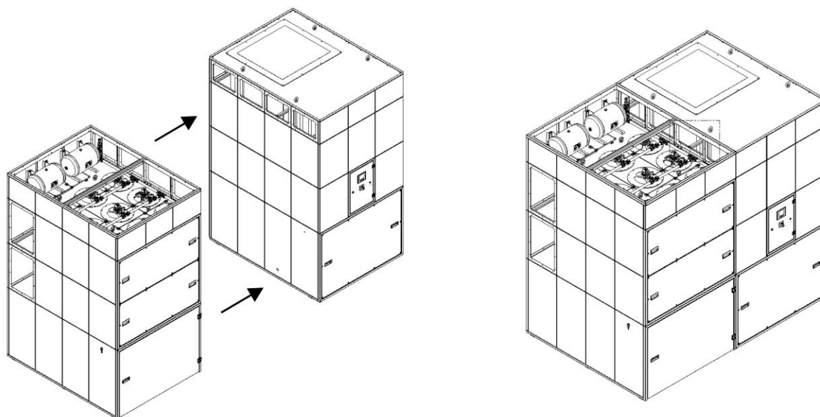
Rys. 20: Połączyć wentylator z filtrem
