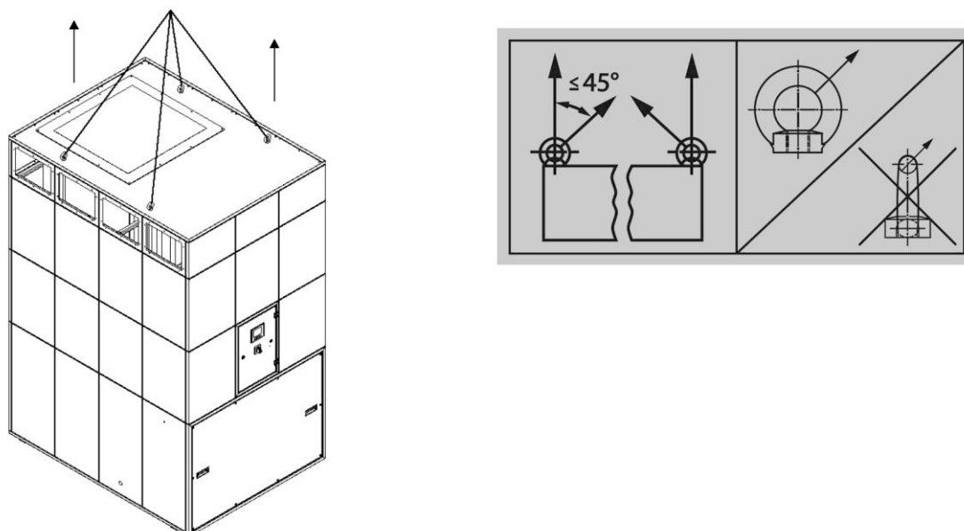
Rys. 10: Podnoszenie modułu wentylatora za pomocą dźwigu
