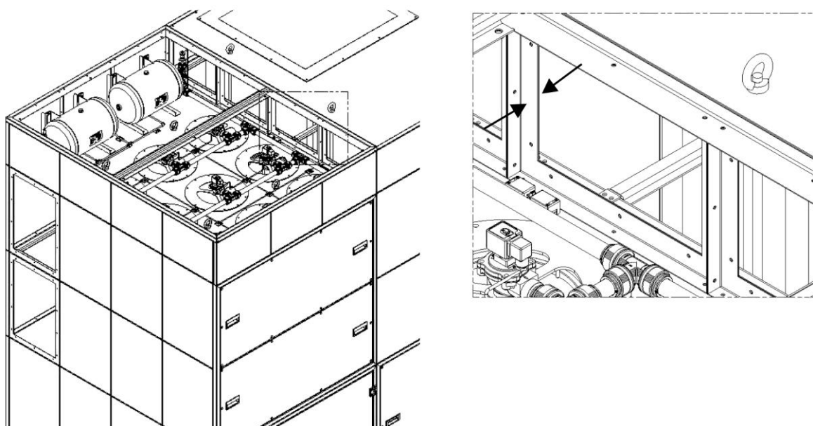
Rys. 21: Łączenie modułu wentylatora z modułem filtra
