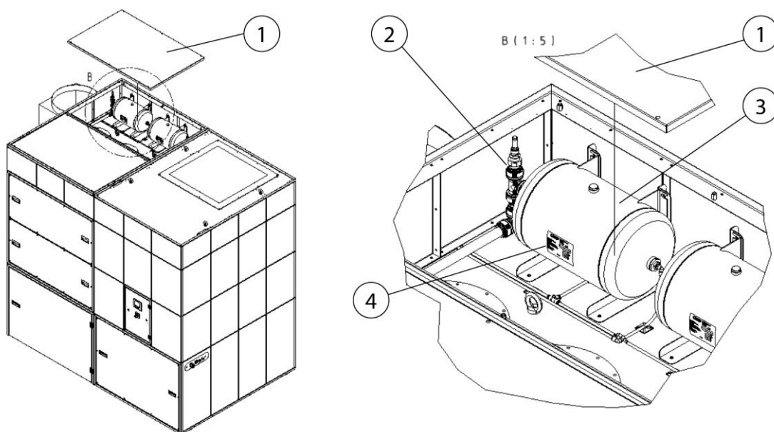
Rys. 74: Dostęp do zbiornika sprężonego powietrza + zawór bezpieczeństwa
