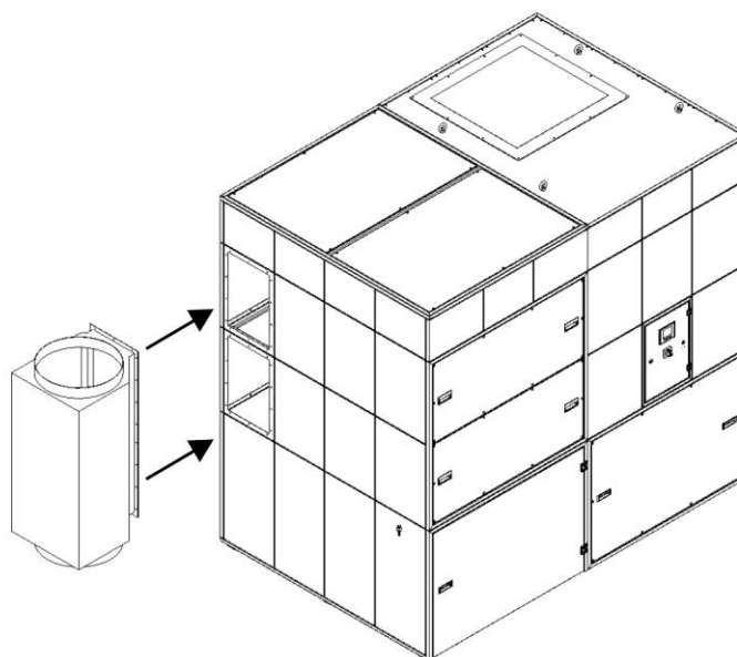
Rys. 26: Montaż skrzynki przyłączeniowej od strony odciągu
