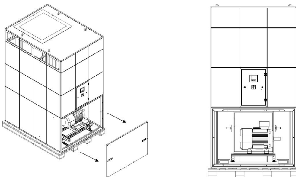
Rys. 9: Otworzyć drzwiczki serwisowe w module wentylatora
