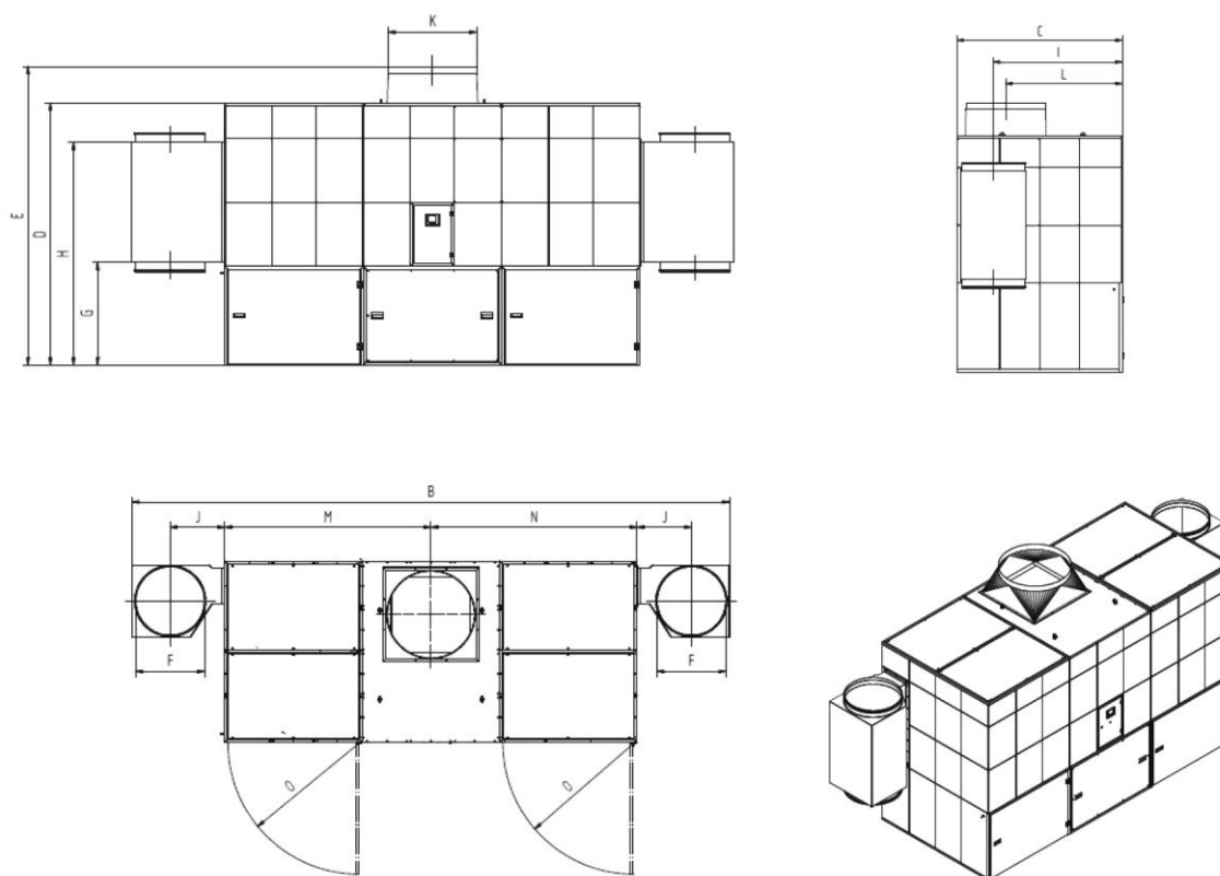
Rys. 79: Karta wymiarów 34200 + 34220
