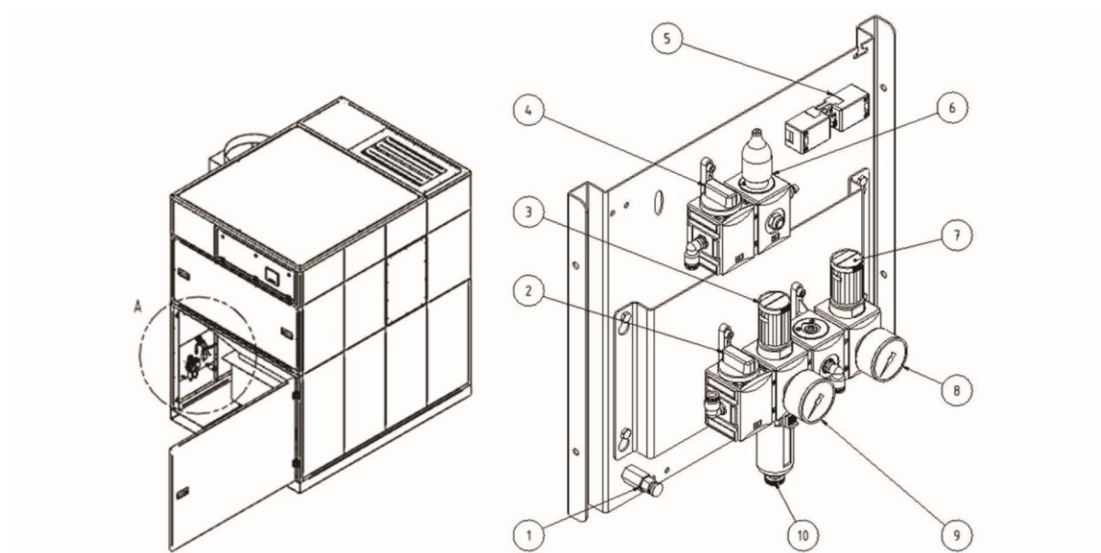
Rys. 27: Jednostka sprężonego powietrza
