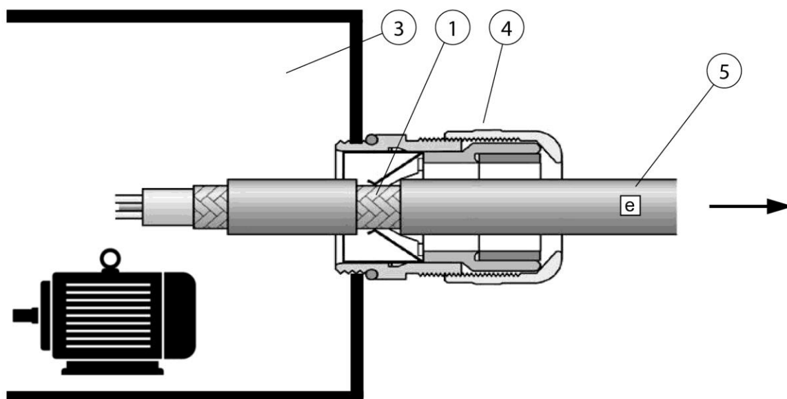
Rys. 37: Podłączenie ekranu przewodu silnika
