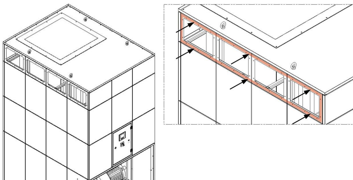
Rys. 12: Przelot czystego powietrza
