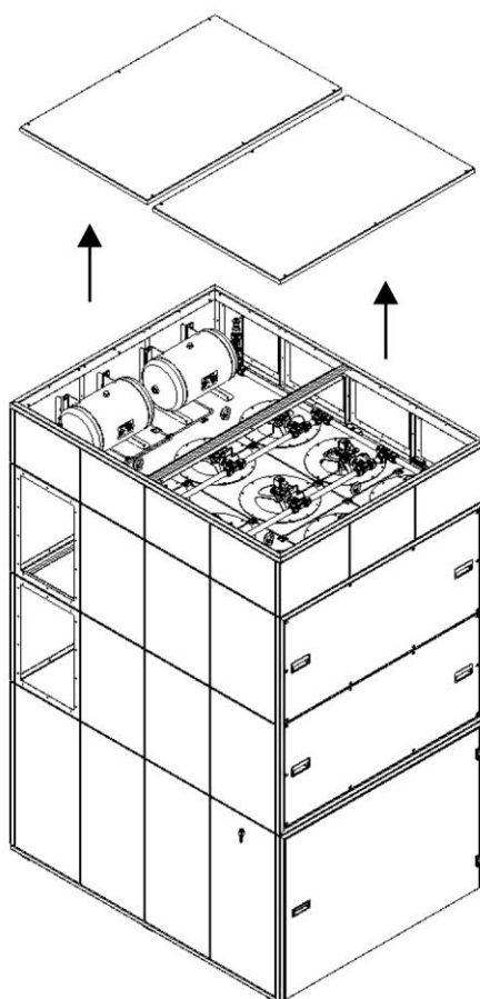
Rys. 17: Zdejmowanie pokryw blaszanych
