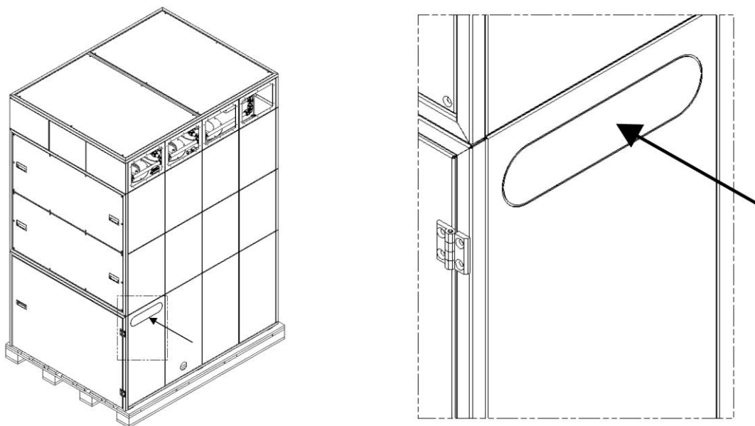
Rys. 13: Blacha frezowana
