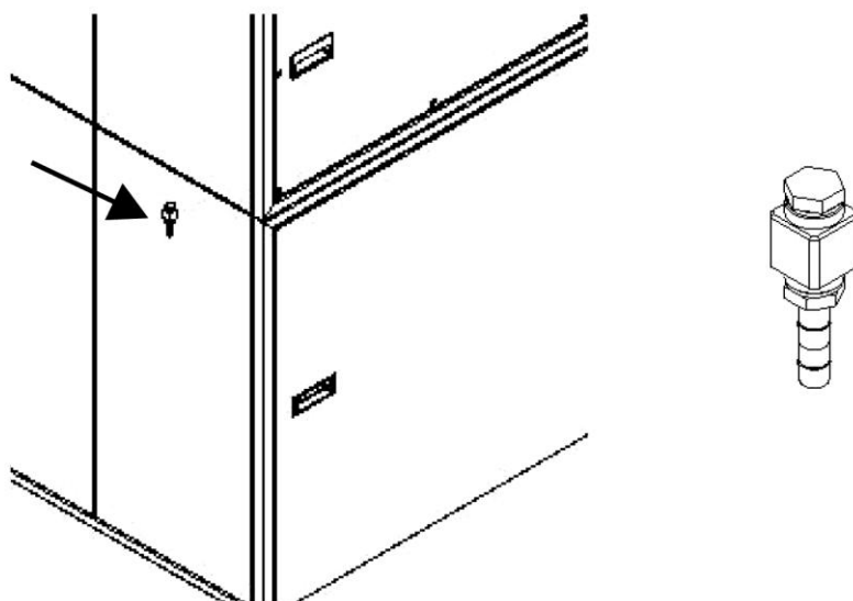
Rys. 28: Przyłącze zasilania sprężonego powietrza
