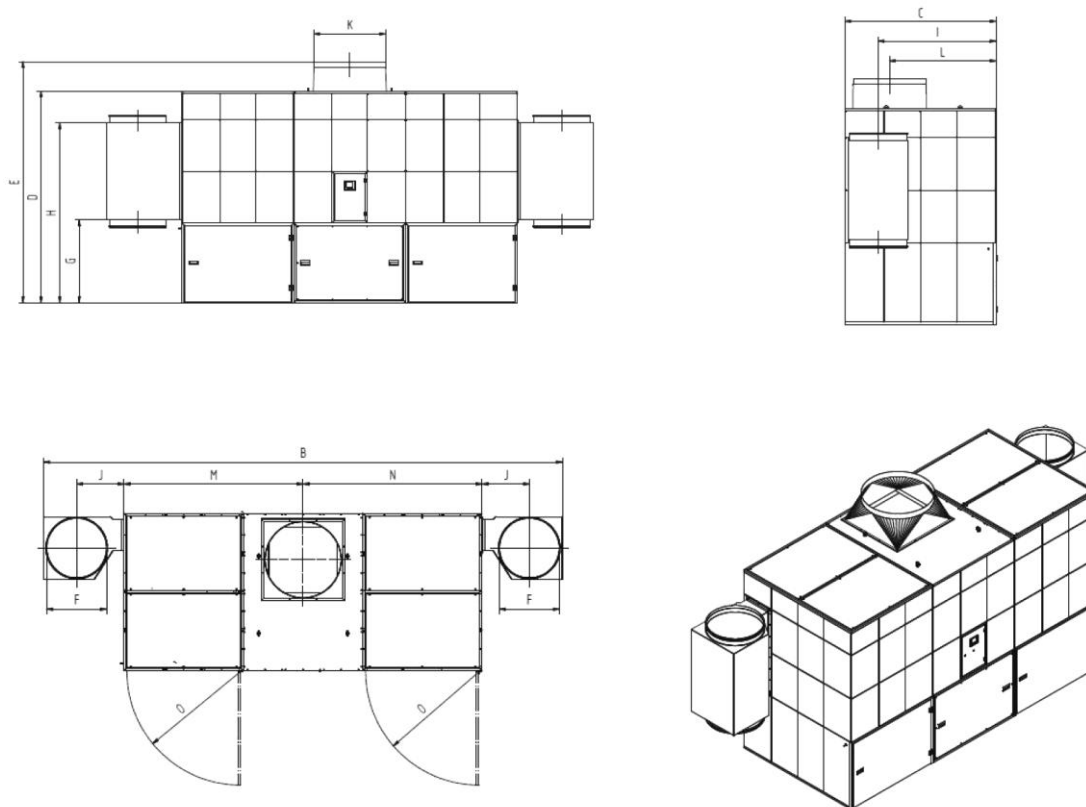
Rys. 78: Karta wymiarowa 34180
