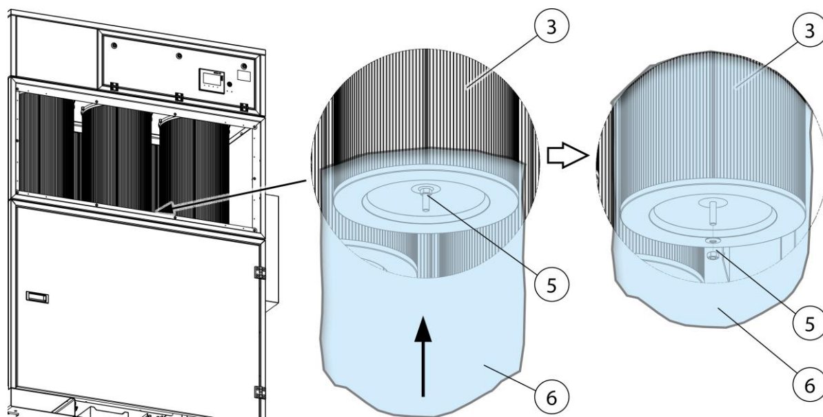
Rys. 62: Wymiana filtra –
