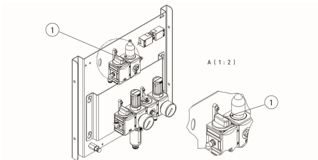
Rys. 55: Zawór pneumatyczny zbiorczego pojemnika na pył
